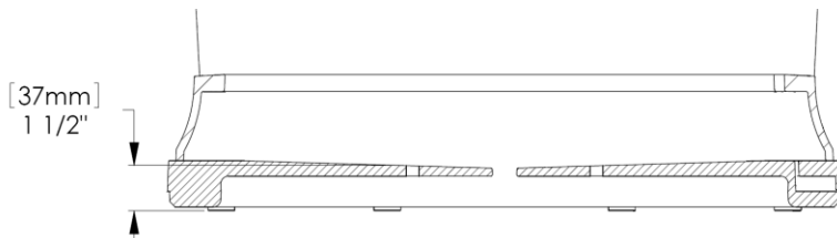
Vue de la base de l'article de coulée
