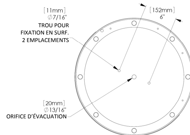
Vue de la base inférieure de coulée
