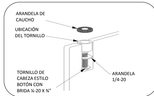
Fig. 1 – Piezas de acoplamiento de las tapas de mesa
